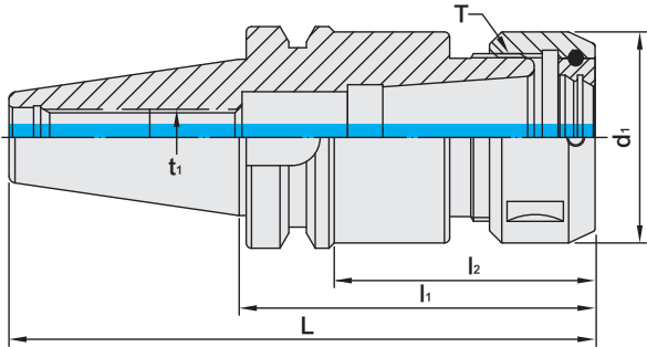
BT / TG 立銑刀夾頭
