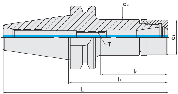
BT / UT 立銑刀夾頭
