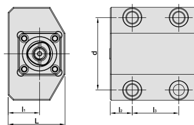
IOTP 一體式內徑刀座 [後拉式]
