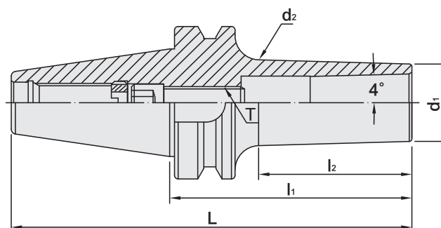
BT / SBL 後拉式立銑刀夾頭
