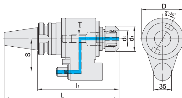
BT / OHER 油路刀把
