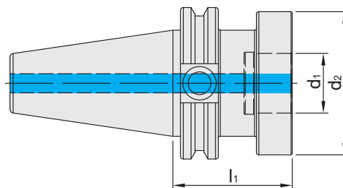
SAF 可調式刀桿本體
