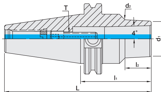
CAT / SBLC 後拉式立銑刀夾頭
