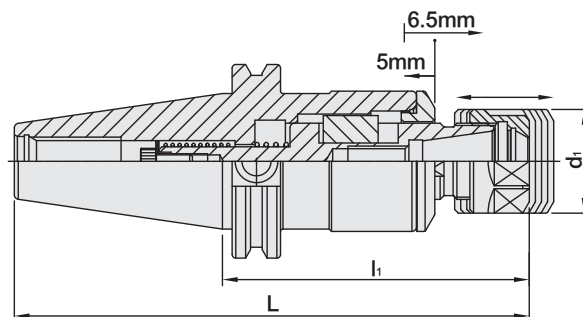
CAT / ETP 伸縮 ER 攻牙器
