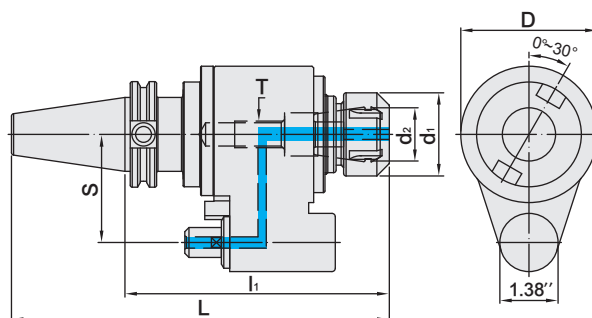
CAT / OHER 油路刀把
