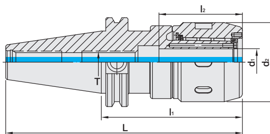
CAT / MLD 直式筒夾 銑床夾頭
