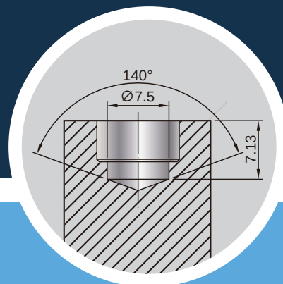
❖ 型式C 預設動平衡 客戶於晶片孔處自行鑽孔 客戶自行安裝晶片
