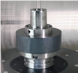
法蘭式油壓刀桿
