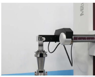
真圓度: 2\mu\text{m}
