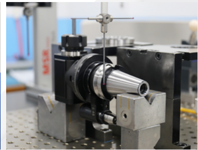
偏擺度: \leq 20\mu\text{m} 傾斜度: \pm 8\mu\text{m}
