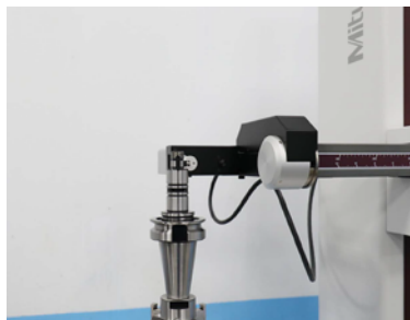
真圓度: 2 \mu\text{m}
